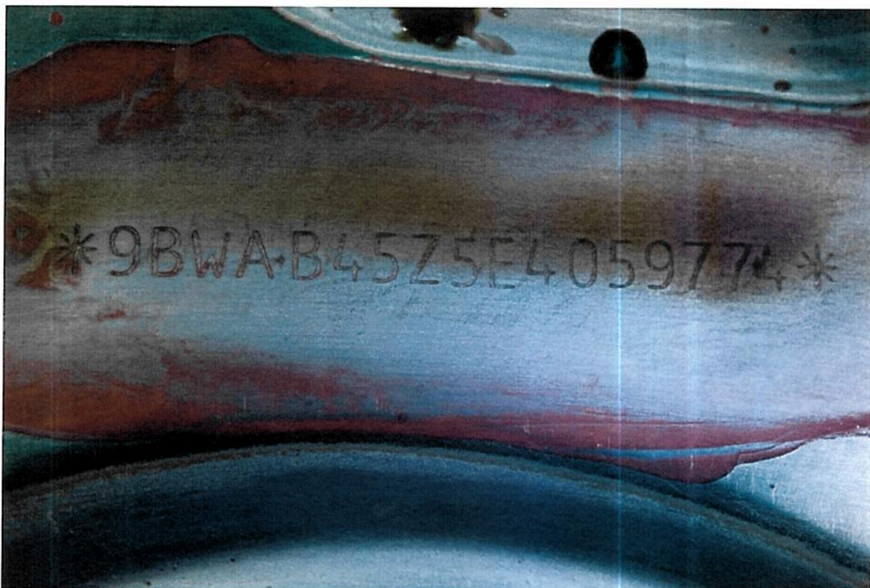
Foto 4. Superfície sede de estampagem do NIV, após exame químico.
