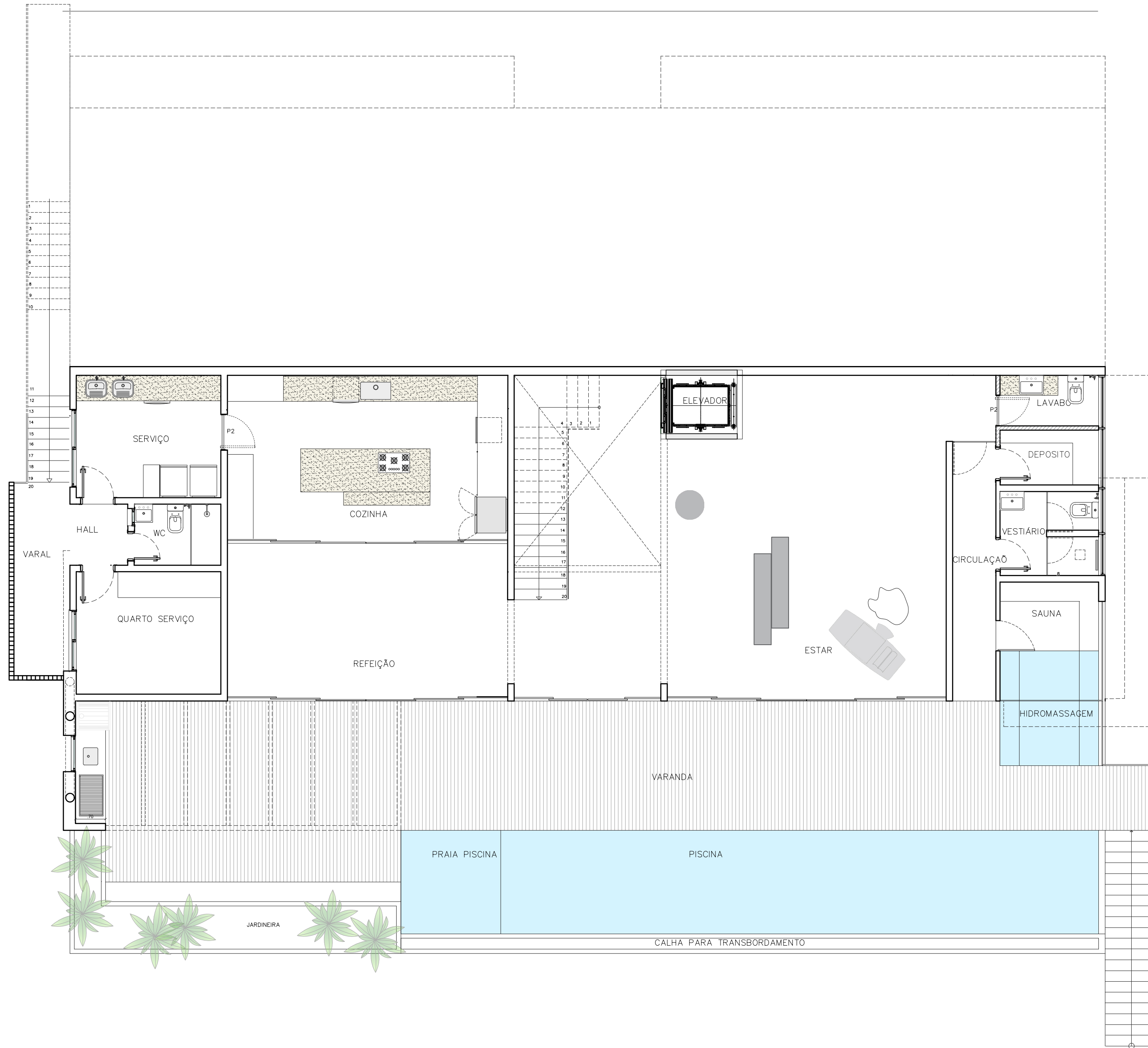
LAYOUT NIVEL INFERIOR ESC. 1:75
