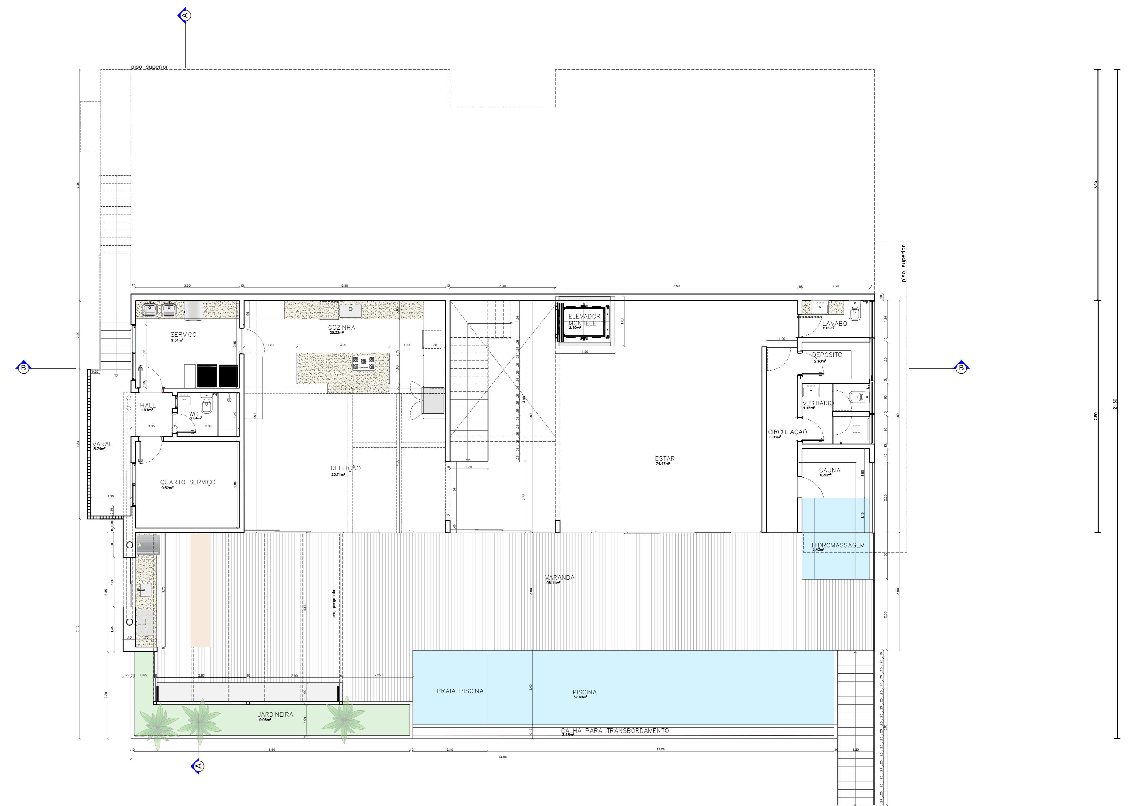
PLANTA BAIXA INFERIOR ESC. 1:75
