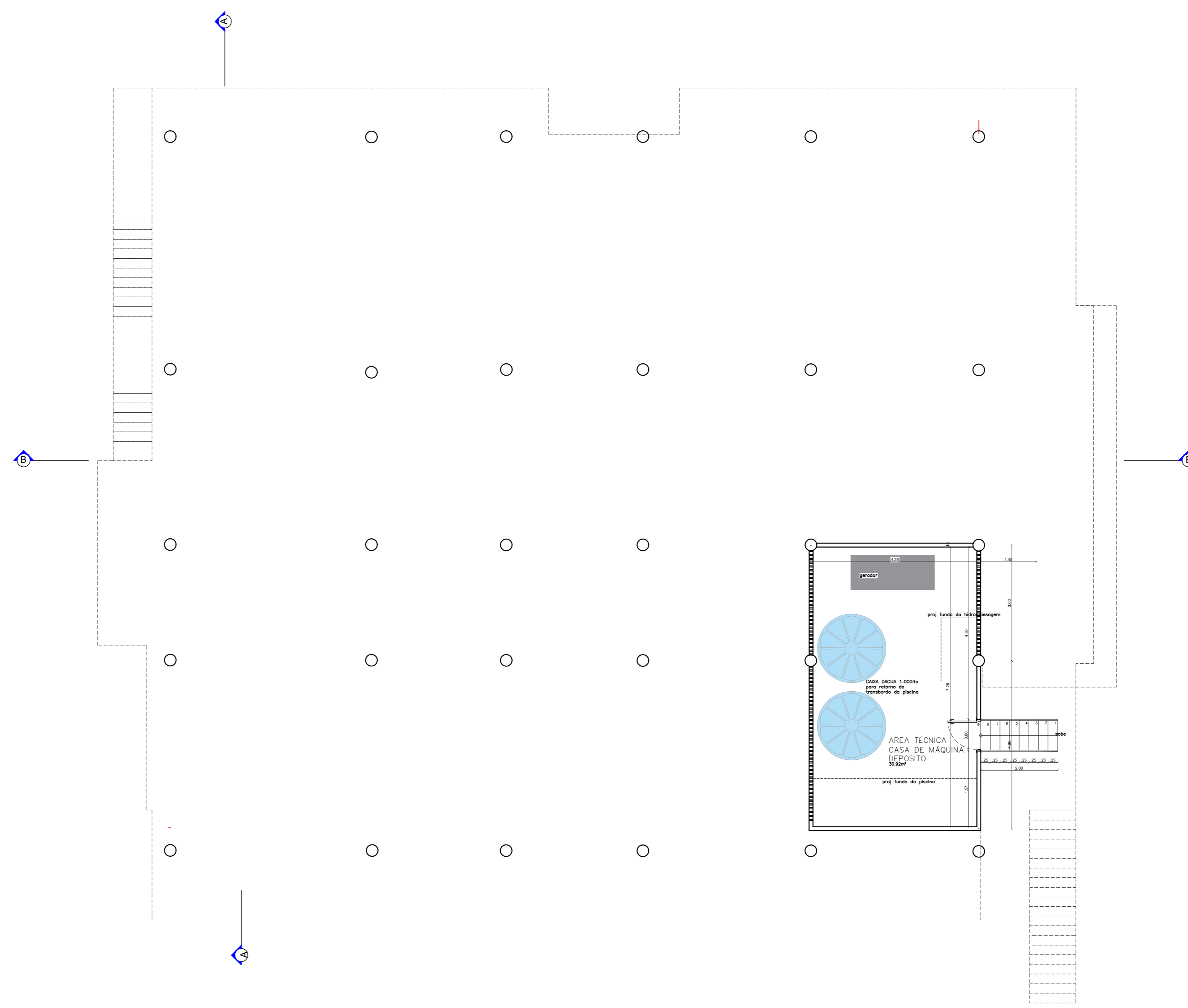
PLANTA BAIXA AREA TECNICA ESC. 1:75
