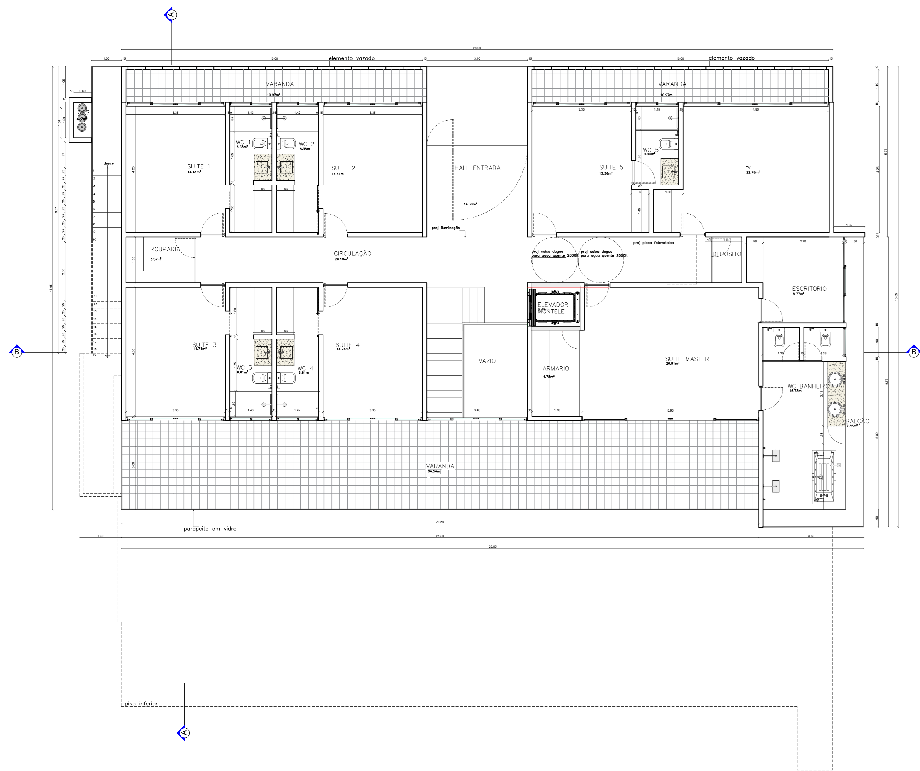
PLANTA BAIXA TERREO ESC. 1:75
