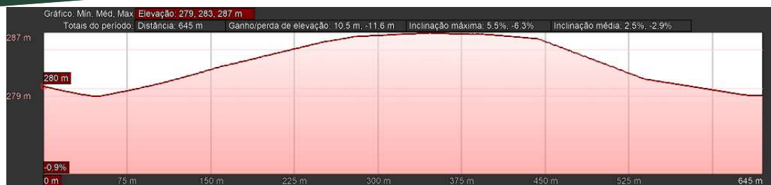
Figura 4 - Perfil de elevação
