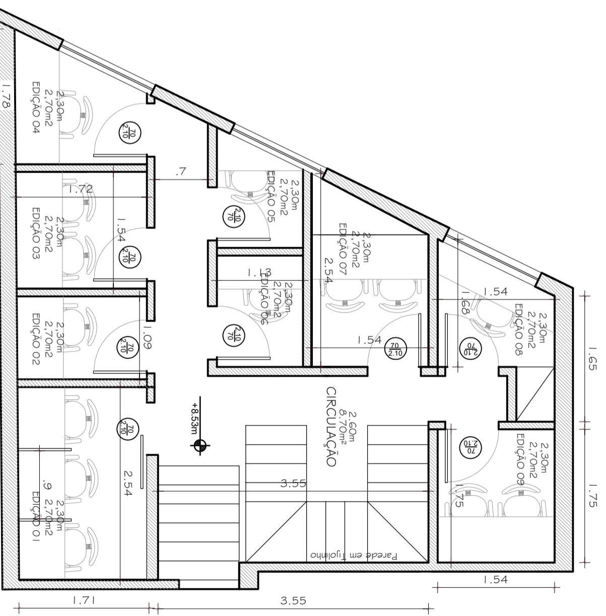
01 PLANTA BAIXA ANEXO - 4º PAVIMENTO ESC. 1/50
