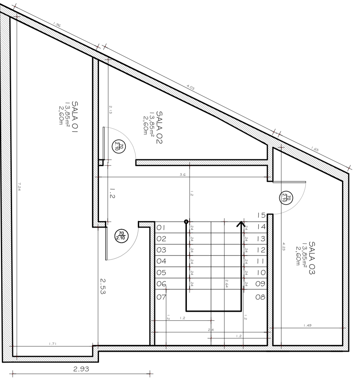
01 PLANTA BAIXA ANEXO PAV 03 ESC. 1/50
