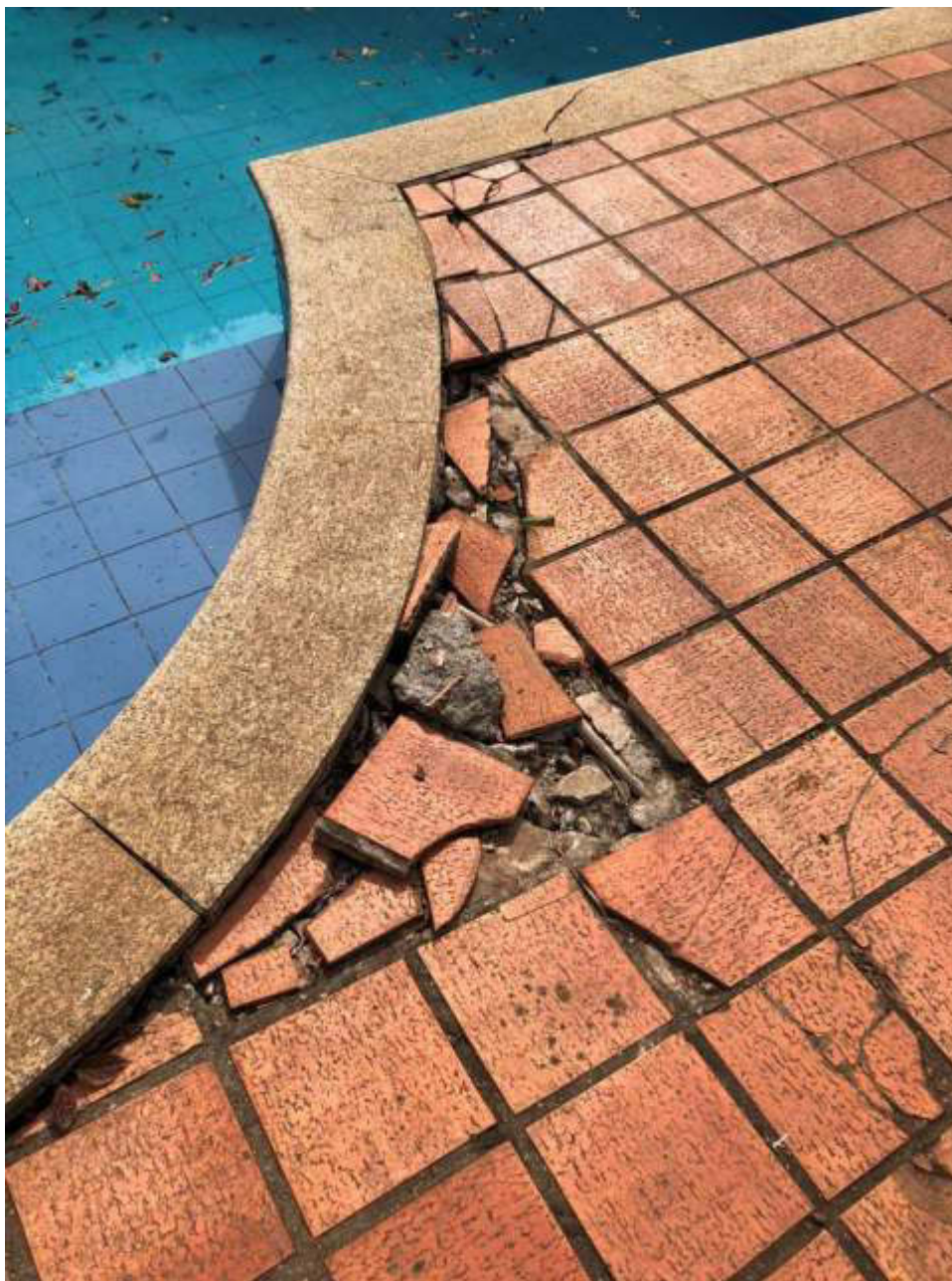
Figura 72: área de piscina com revestimento quebrado
