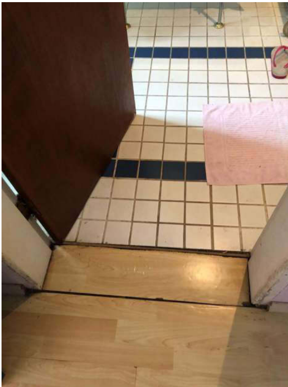
Figura 42: suíte 1 - marcas de estufamento do assoalho de madeira
