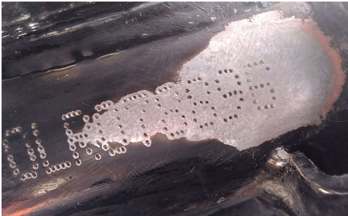
Foto 3: Mostra porção final da gravação do NIV no chassi com sinais de adulteração.
