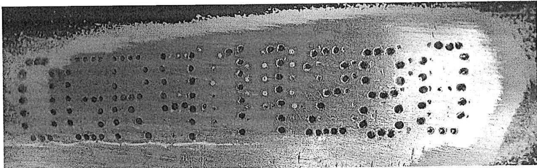
Foto 2: Mostra gravação subjacente do NIV do Chassi. Final mais provável GR204826
